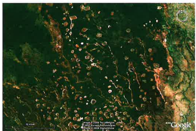
Figuur 15. Zwerm van pannen met gemiddelde doormeter tussen 600 meter en 1,25 kilometer in rode laterietbodem (ferralsol) op laagplateau in tertiaire fluviaatiele-lacustriene zanden en kleien met ongeordend anastomoserend drainagepatroon in de kustvlakte net ten zuiden van de Zambezi rivier in Mozambique (E 35°35' S 18°18') (bron Google Earth).
