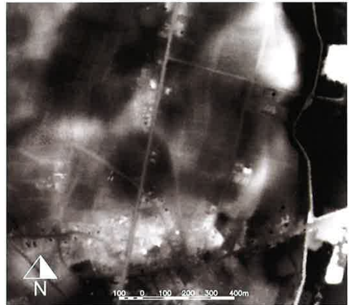
Figuur 10. Panchromatisch beeld van over elkaar groeiende windkuilen net ten noorden van Ophoven, waarbij de centraal gelegen zwarte (dus laaggelegen) ronde depressies jonger zijn dan de zowel grotere als kleinere meer grijze vormen.
