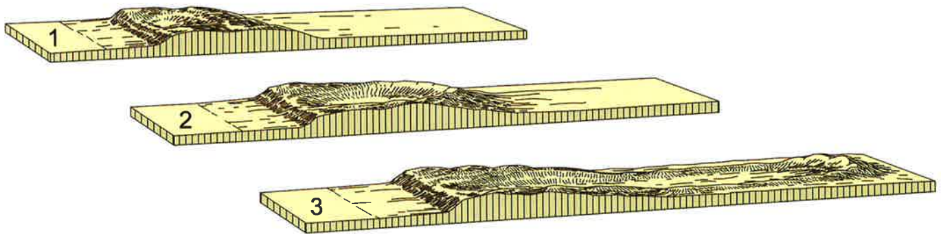
Figuur 17a. Evoluteschema van windkuil tot boogduin (paraboolduin), naar van Houten (1939) in Escher (1962), aangepast aan het microreliëf van de Vlakte van Bocholt.
